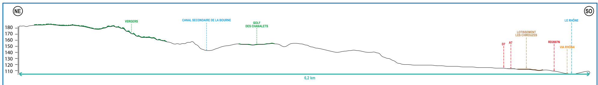
Coupe topographique
